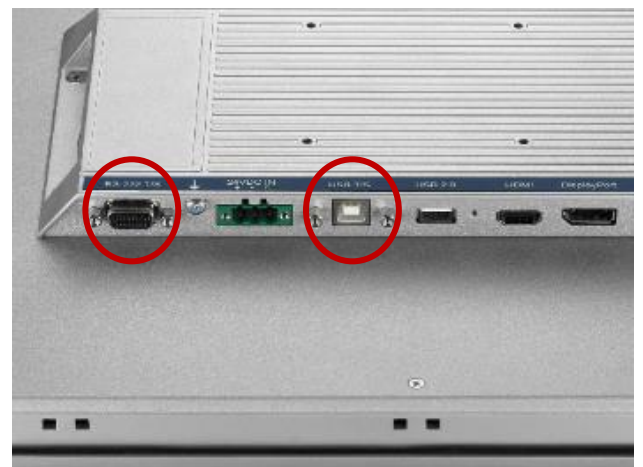
RS-232 / USB
